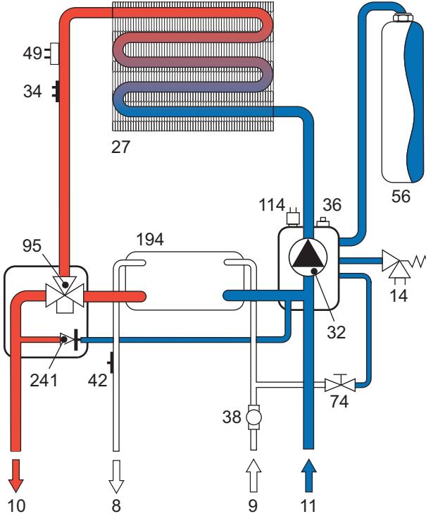
рис. 21 - Отопительный контур
