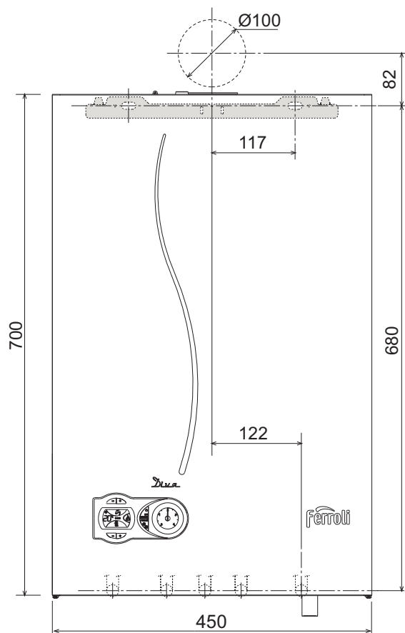
рис. 16 - Вид спереди
