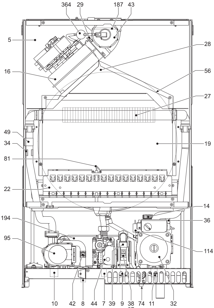
рис. 20 - Общий вид
