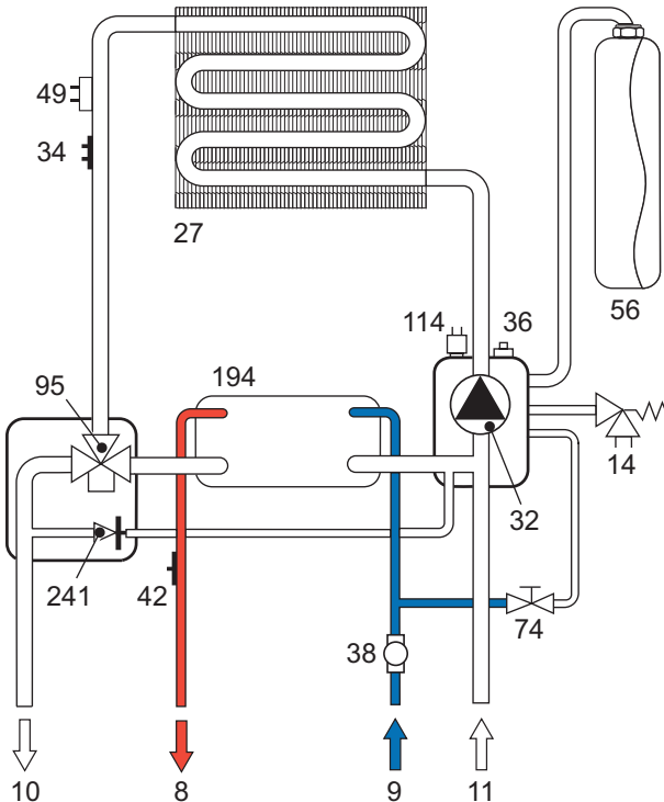
рис. 22 - Контур ГВС
